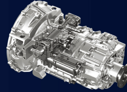
ZF 6단 수동변속기
