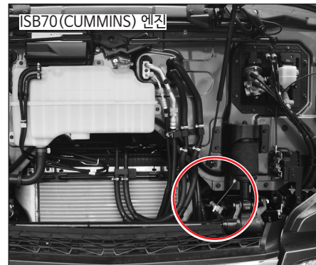
4)ISB70(CUMMINS) 엔진 : 앞 점검 판넬을 당겨서 열면 라디에이터 오른쪽에 게이지가 있습니다.
