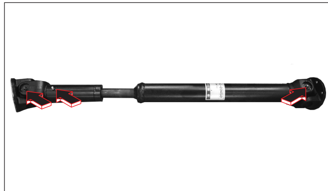
7) P.T.O 드라이브 샤프트
