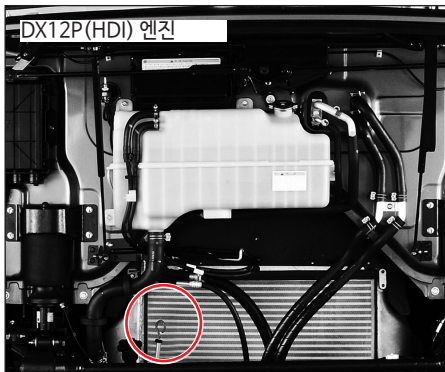
3)DX12P(HDI) 엔진 :앞 점검 판넬을 당겨서 열면 라디에이터 앞쪽에 게이지가 있습니다.
