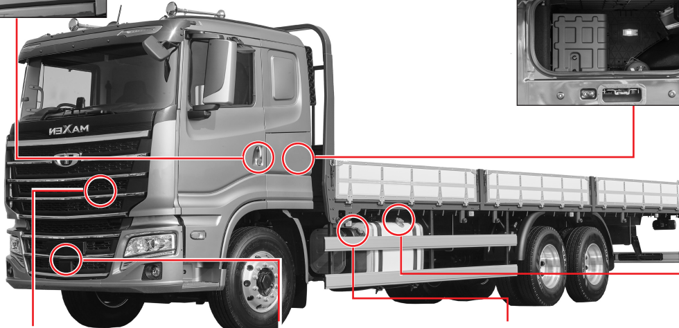
앞 점검판넬 고정해제 레버
