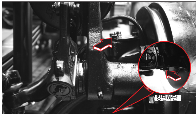
1) 킹핀
