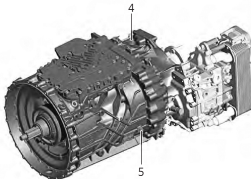
ZF TRAXON 자동변속기 + 인타더
