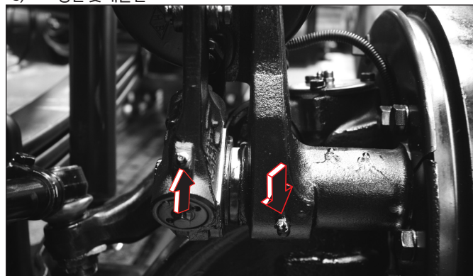
4) 프런트 챔버브라켓 및 슬랙어저스트(드럼 브레이크 적용차량)
