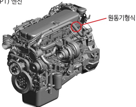
CURSOR 13(FPT) 엔진
