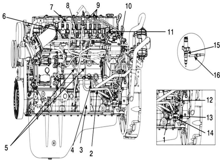
ISB70(CUMMINS)엔진
