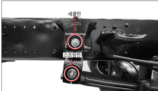
2) 스프링핀 및 새클핀
