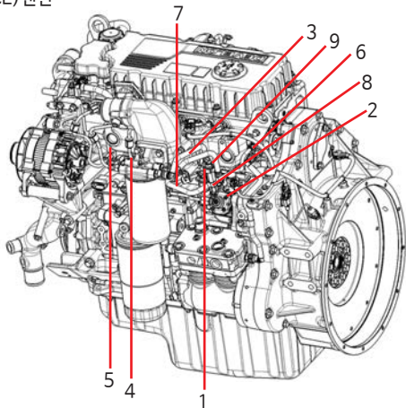
DX05(HCE)엔진
