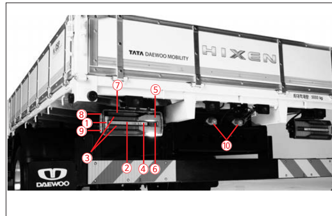
후방 램프
