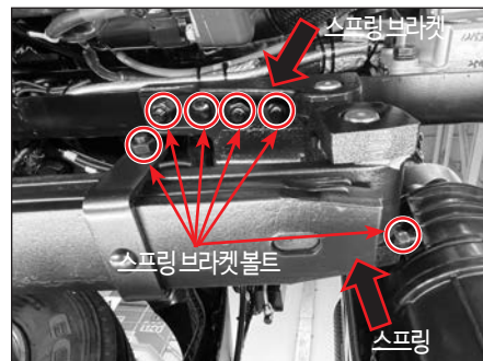
뒤쪽 스프링 브라켓 볼트
