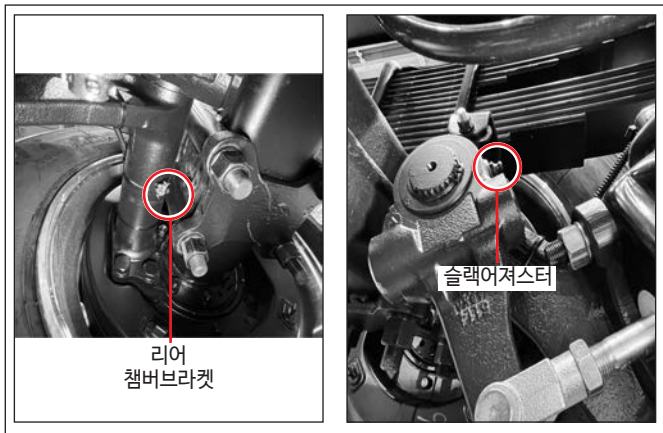
4) 리어 챔버브라켓 및 슬랙어저스터
