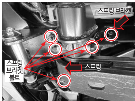
앞쪽 스프링 브라켓 볼트
