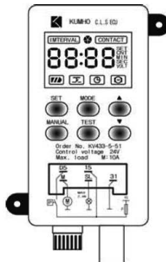
콘트롤 유니트(콘트롤러)
