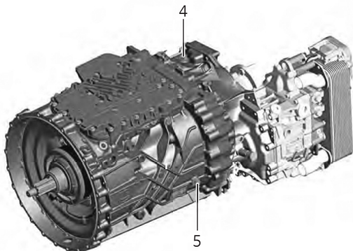
ZF TRAXON 자동변속기 + 인터더
